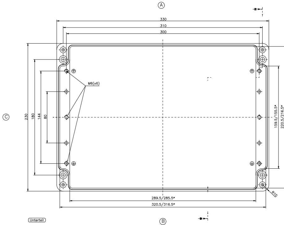
(Unterteil)
